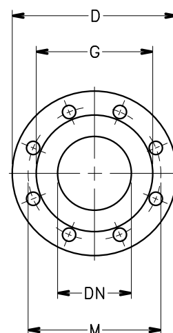
ФЛАНЦЫ НАСОСА
