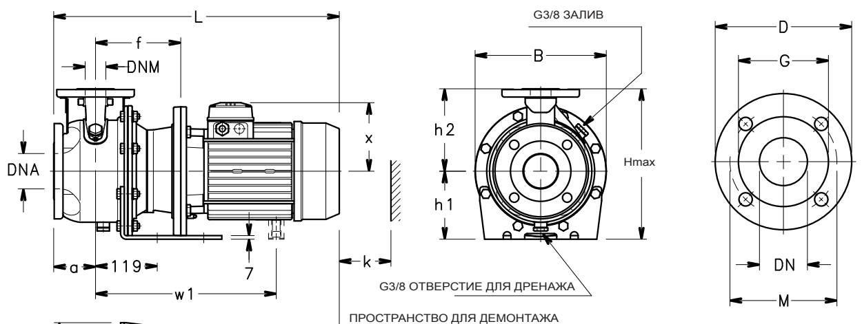
SHS С ОПОРОЙ НАСОСА ДВИГАТЕЛИ МОЩНОСТЬЮ ДО 7,5 кВт
