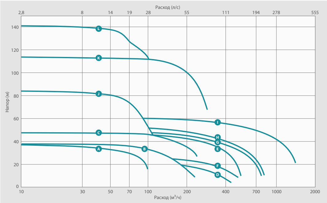
Данные кривые представлены только для сравнения. Точные характеристики по расходу и напору указаны в технических данных.
