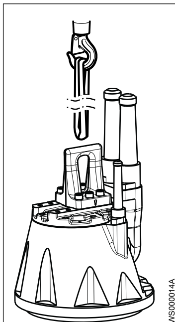
Рис. 5: Блоки привода 805–998
