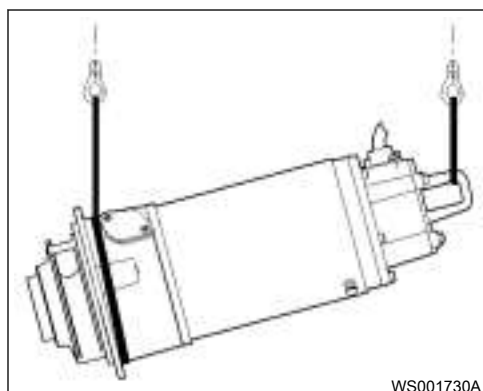
Рис. 74: Поднимите с помощью грузоподъемного стропа и подъемной рукоятки
