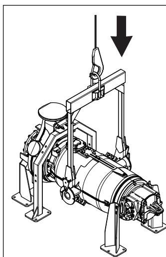
Рис. 76: Опускание подъемника
