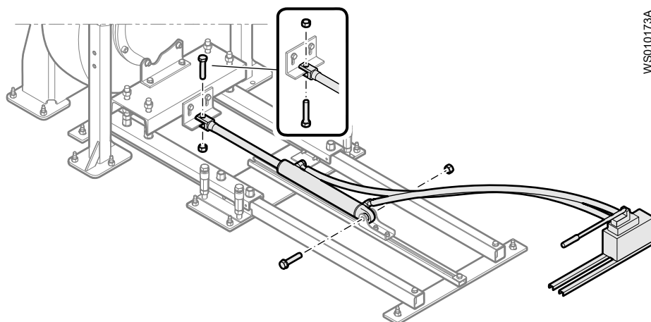
Рис. 35: Установка ручного насоса. (Насос не показан.)
