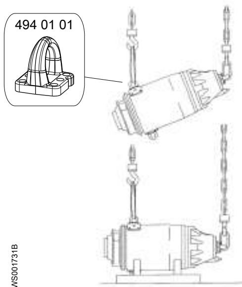
Рис. 75: Поднимите с помощью кронштейна с подъемным ушком 494 01 01 и подъемной рукоятки на верхней части привода
