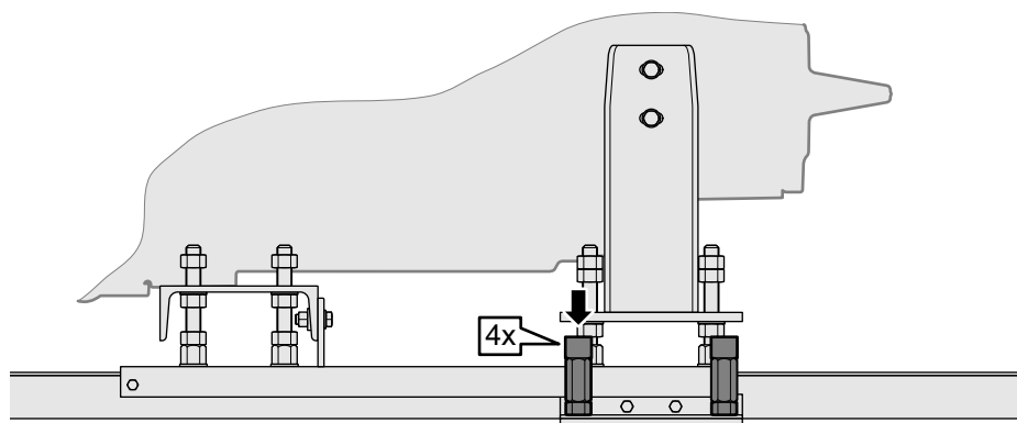
Рис. 89: Опускание внешних опор
