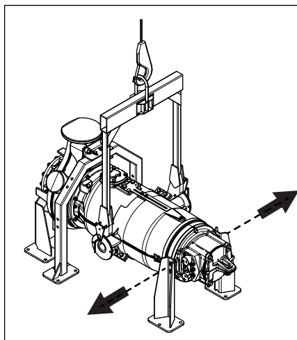
Рис. 78: Снятие с верхней части насоса поддерживающих опор
