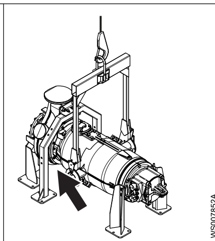
Рис. 79: Отсоединение привода от гидравлического блока
