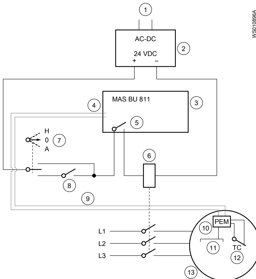
Рис. 47: Тепловые контакты или терморезисторы подключены к РЕМ
