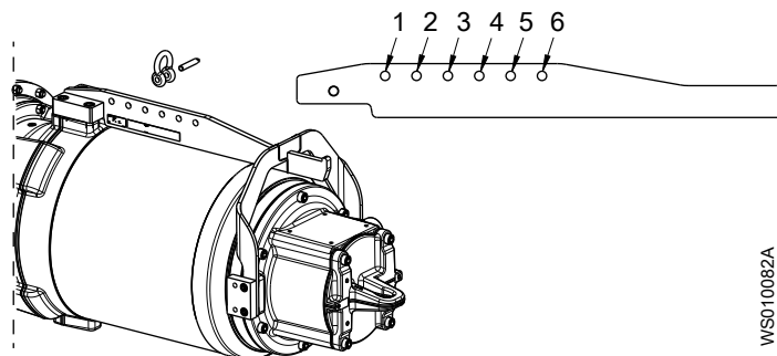
Рис. 81: Установка скобы
