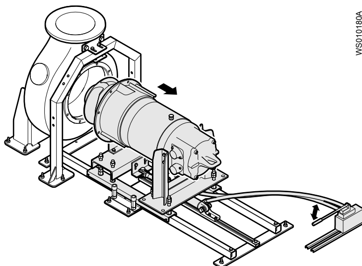
Рис. 92: Передвижение блока привода при помощи ручного насоса
