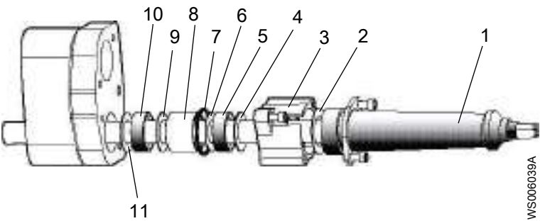
Рис. 48: Блоки привода 605-776
