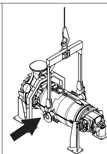
Рис. 77: Проверка стопорного штифта
