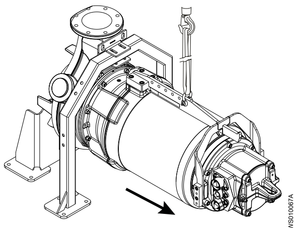
Рис. 85: Демонтаж привода
