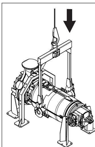
Рис. 76: Опускание подъемника
