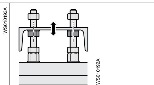
Рис. 96: Регулировка по вертикали
