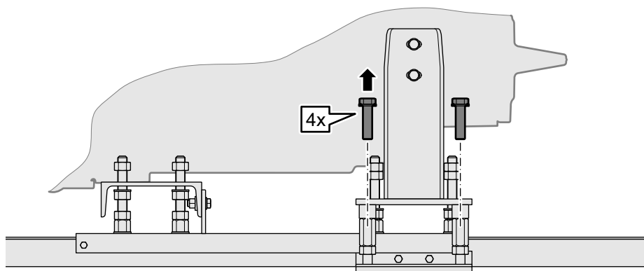
Рис. 87: Снятие болтов
