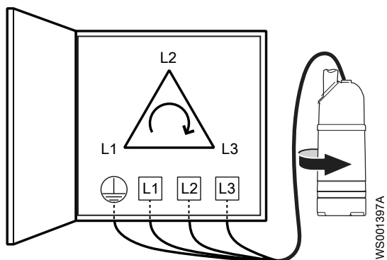
Рис. 5: Включите насос
