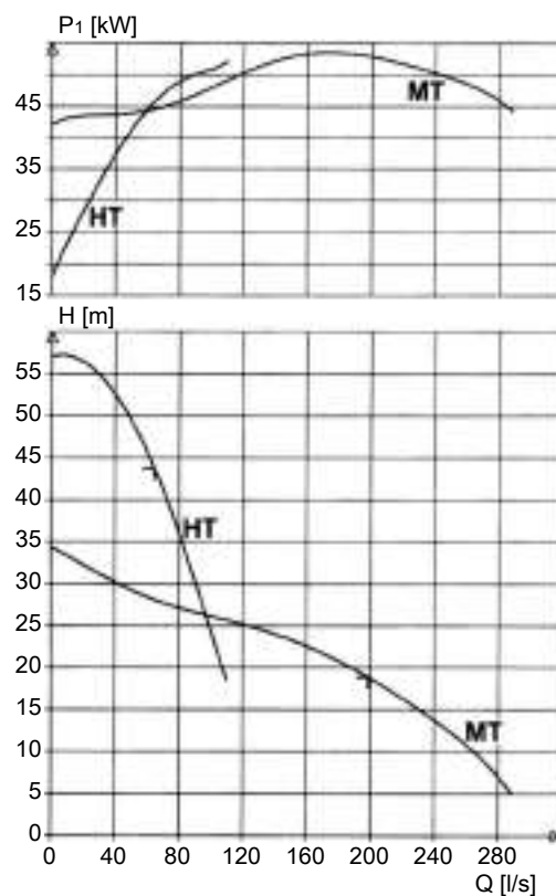
Рис. 7: 50 Гц, 1 470 об/мин
