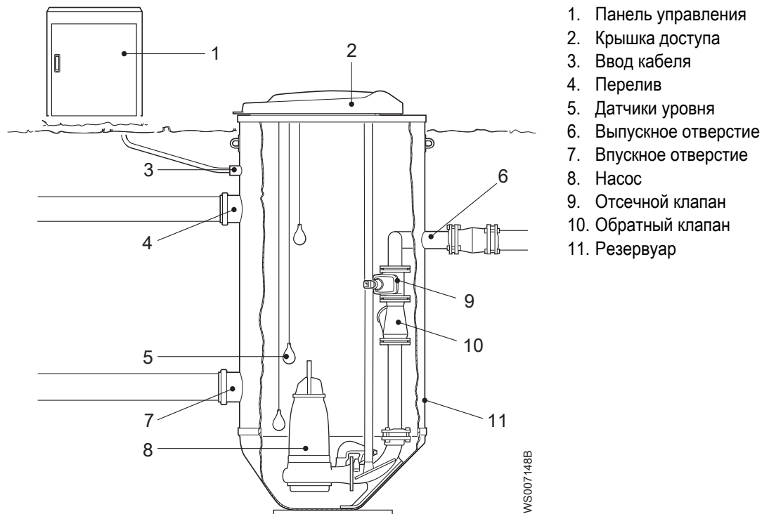
Рис. 4: Пример установки
