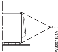
Рис. 3: Подъемные проушины для стропы
