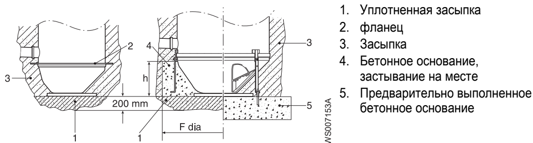
Рис. 8: Конструкция основания колодца
