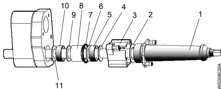
Рис. 10: Блоки привода 605–675
