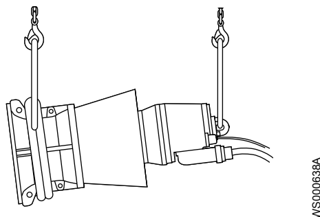
Рис. 30: Поднимите агрегат для ремонта. Показан типовой агрегат.
