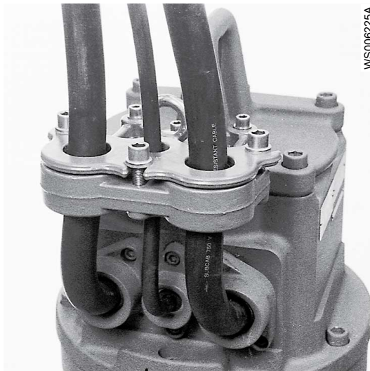
Рис. 12: Держатель кабеля. В насосах с MAS 801 нет вспомогательного кабеля.
