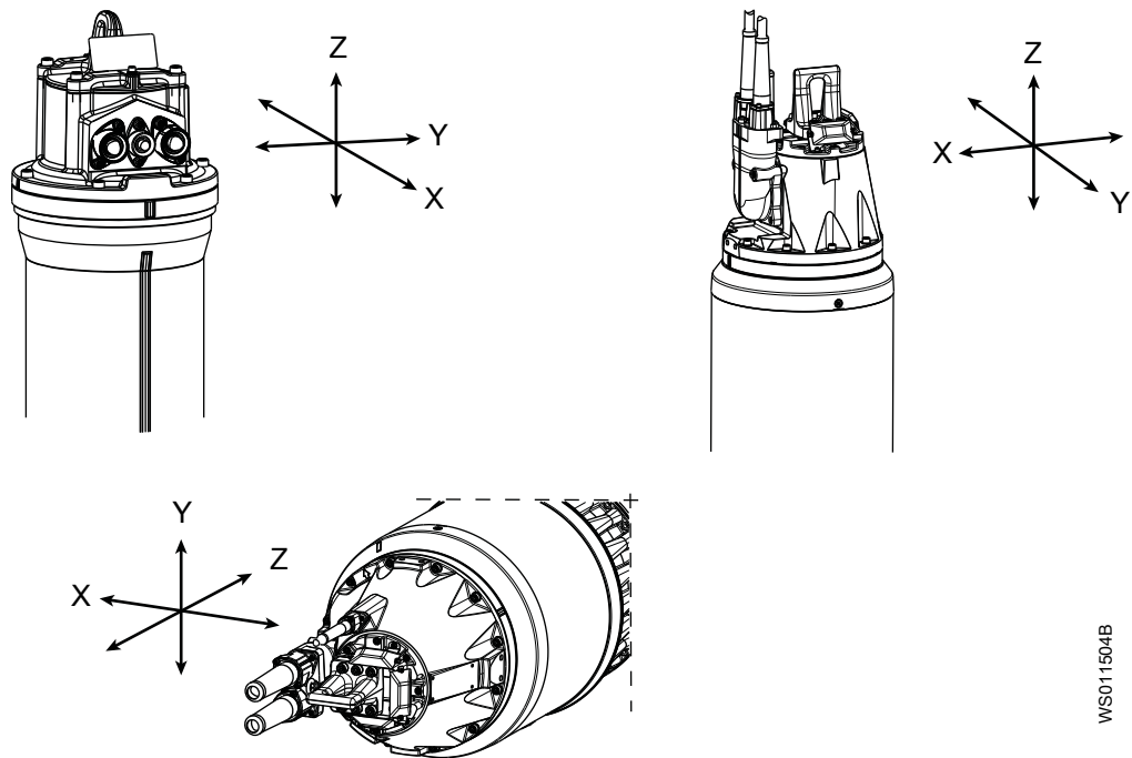
Рис. 4: Направление вибрации по отношению к насосу
