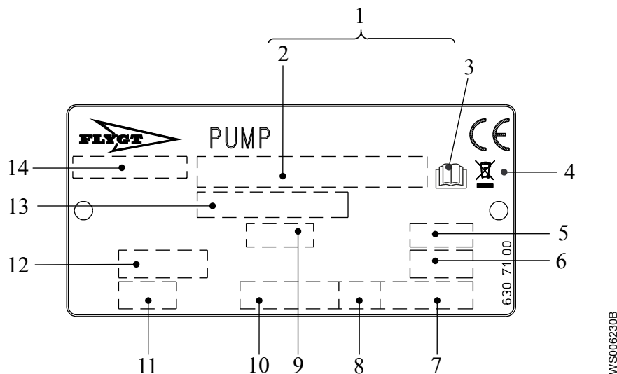
Рис. 5: Табличка для приводного блока начиная с 990101
